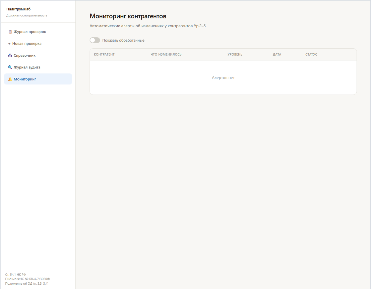
Раздел «Мониторинг»
