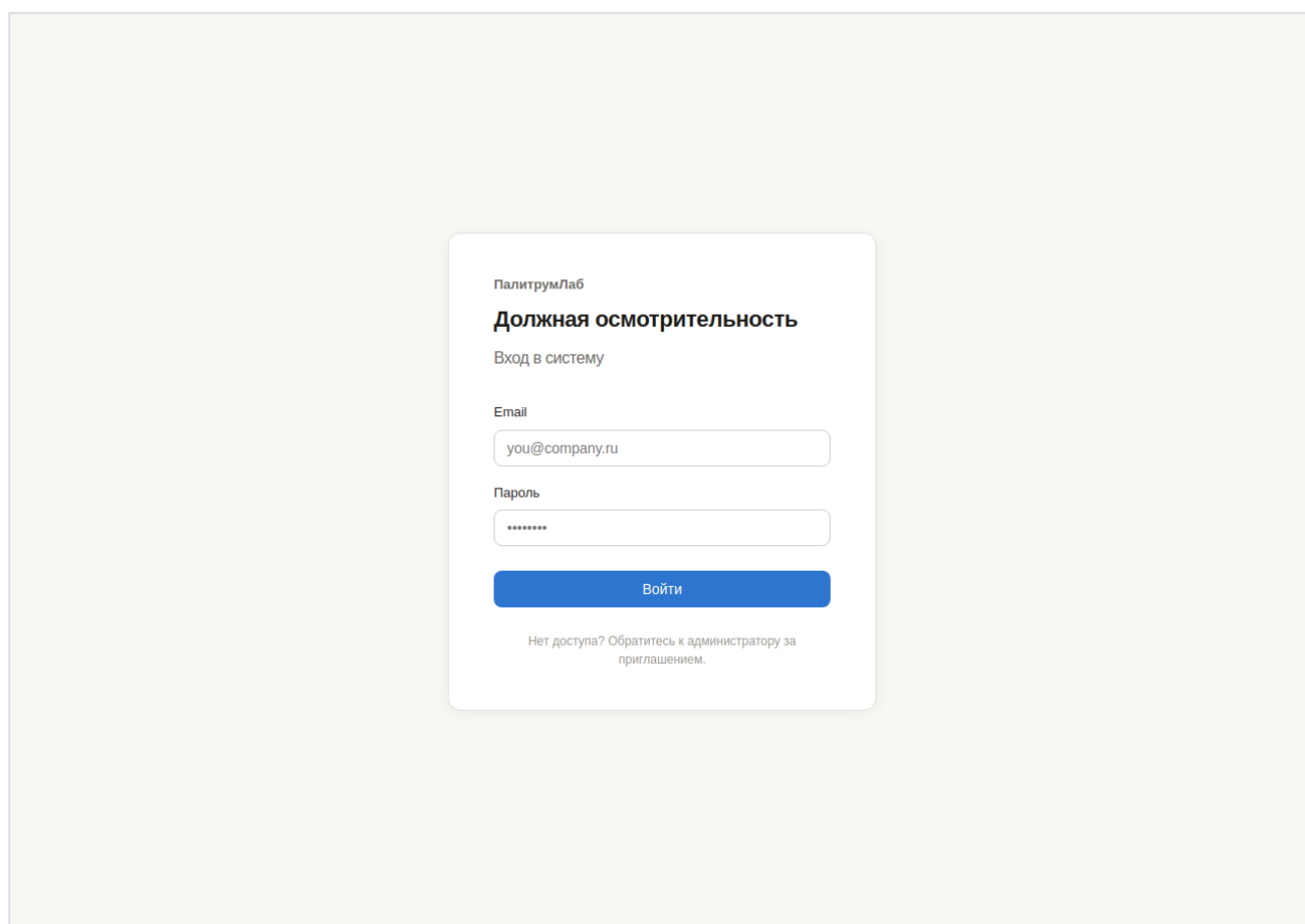
Экран входа
